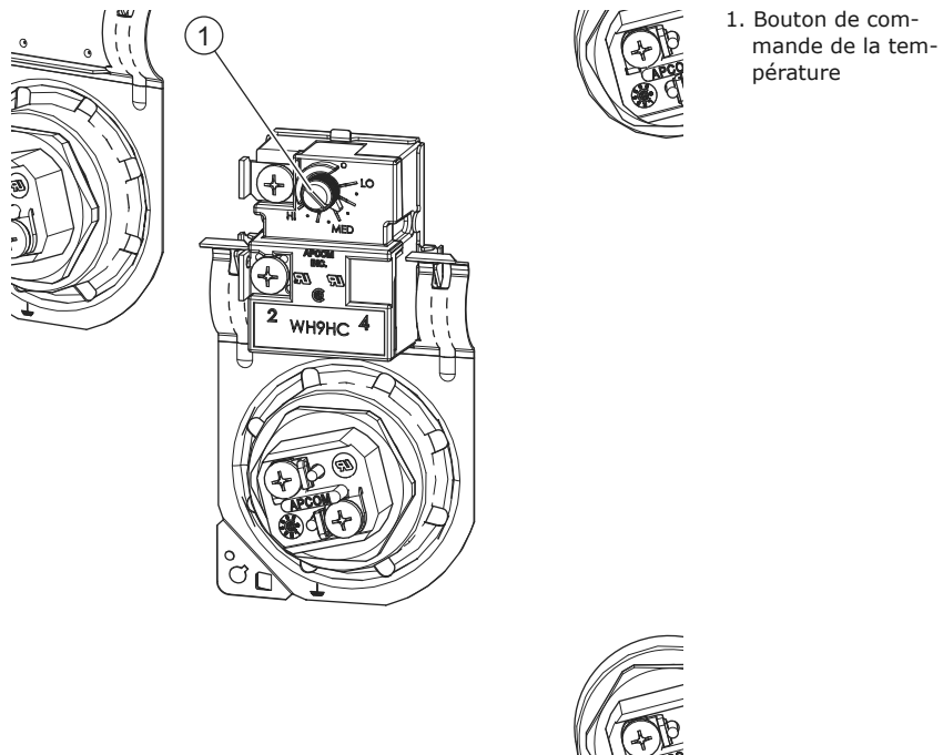
Illustration : Composants de commande
