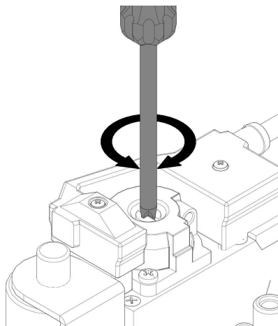
Illustration : SGS 80-120 - Réglage CO 2 (charge partielle)
