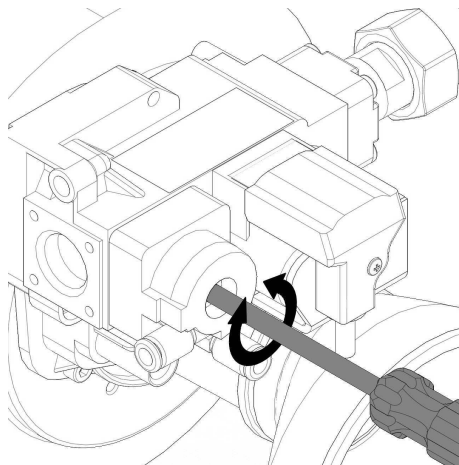
Illustration : SGS 28-60 - Réglage CO 2 (charge partielle)
