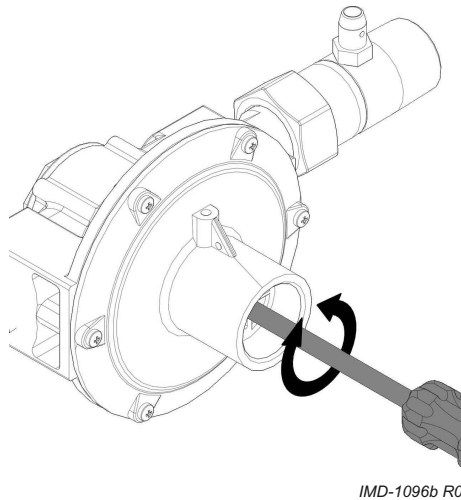
Afb. De gasblokdruk afstellen
