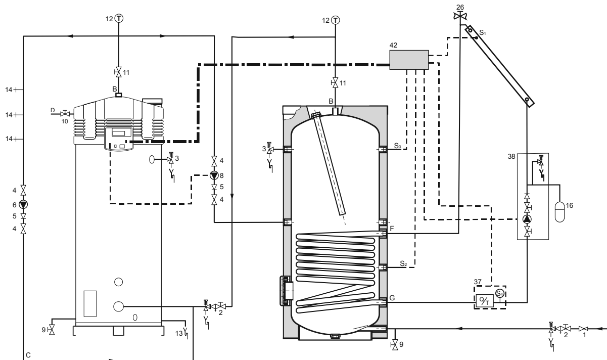
Afb. Installatieschema
