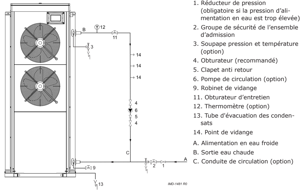
Illustration : Schéma d'installation
