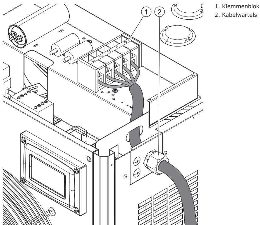
Afb. Aansluitblok
