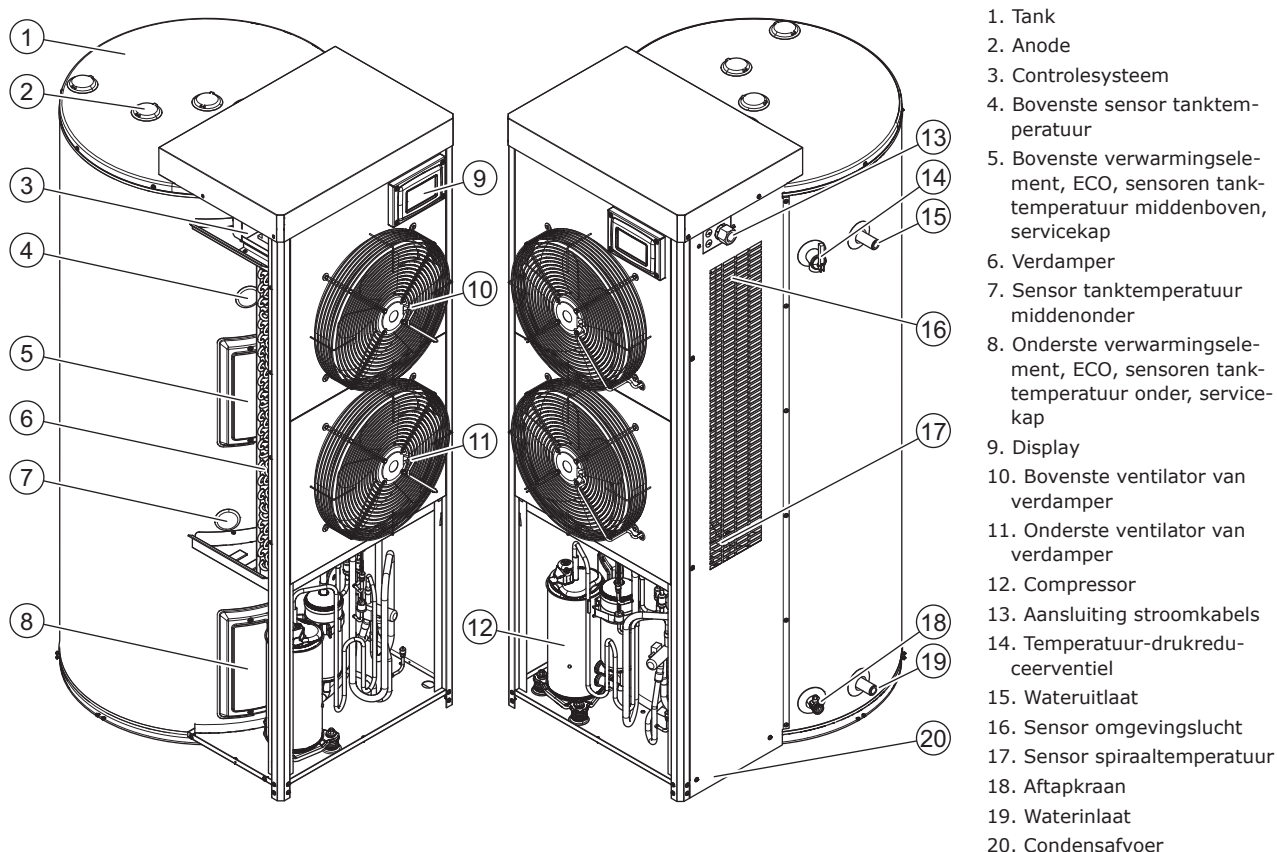
Afb. Onderdelen van de boiler
