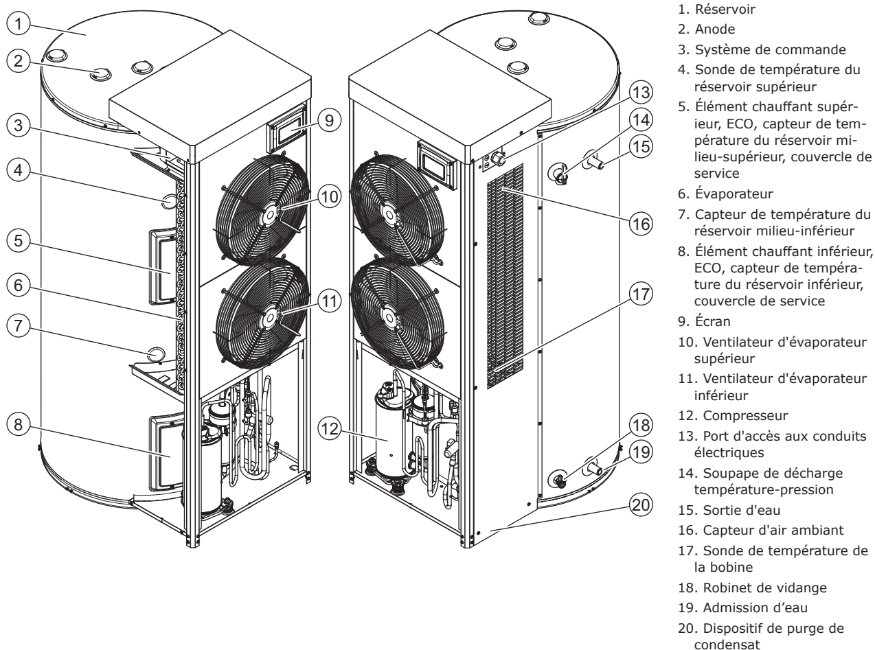
Fig. Composants du chauffe-eau
