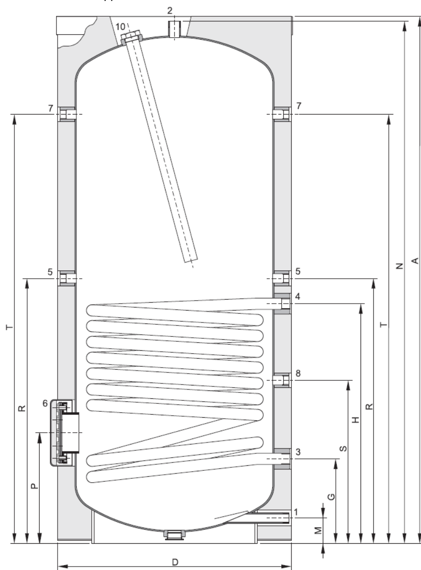
Vue de frontale des appareils
