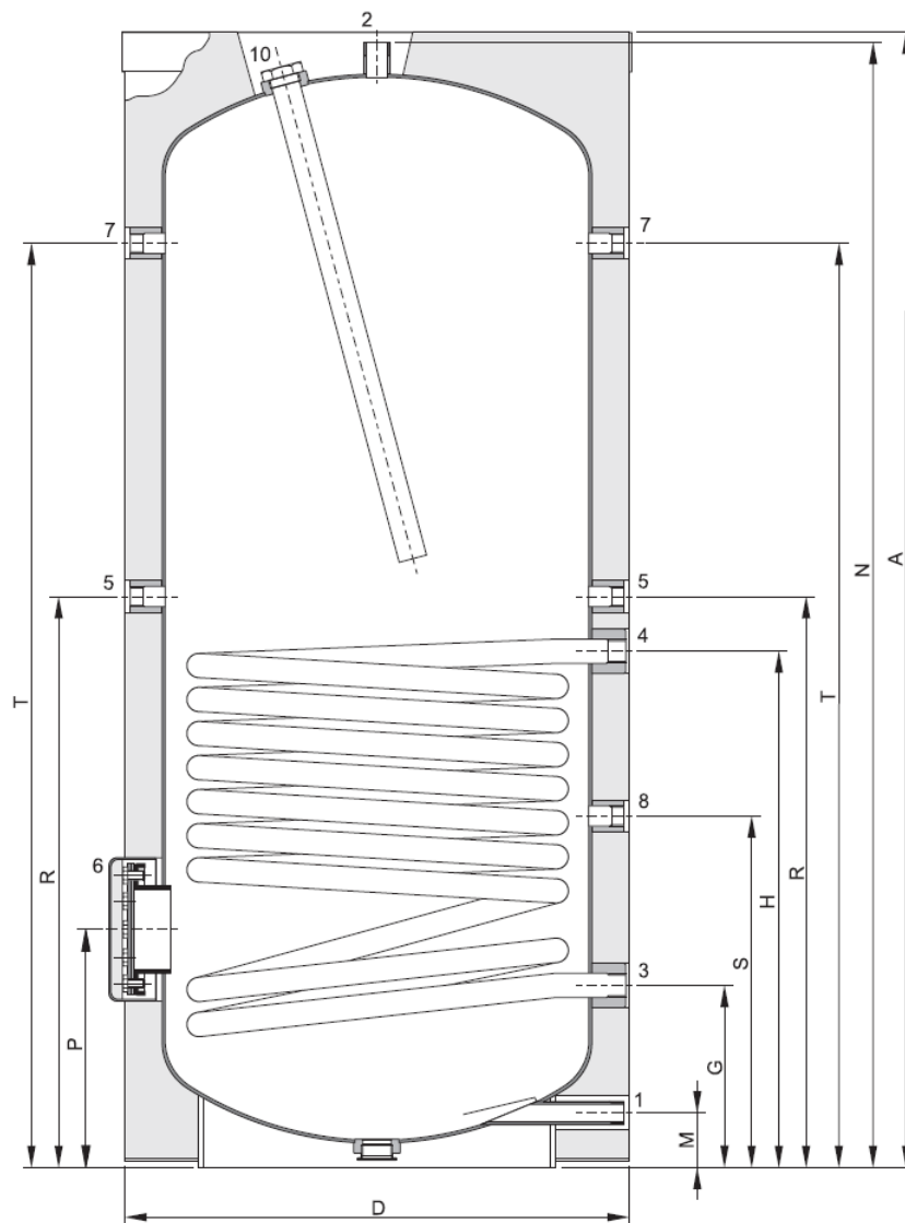
Vooraanzicht doorsnede toestel
