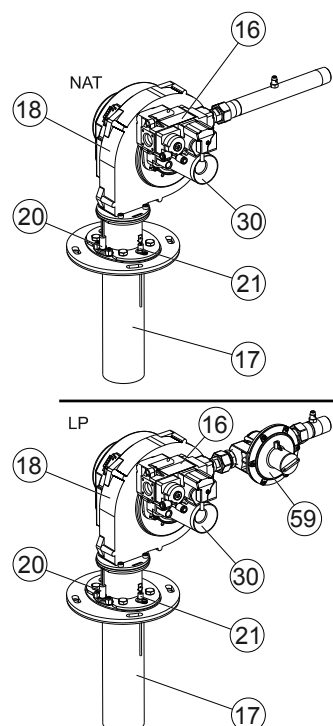
Fig. Calentador de agua BFC 28, 30, 50, 60
