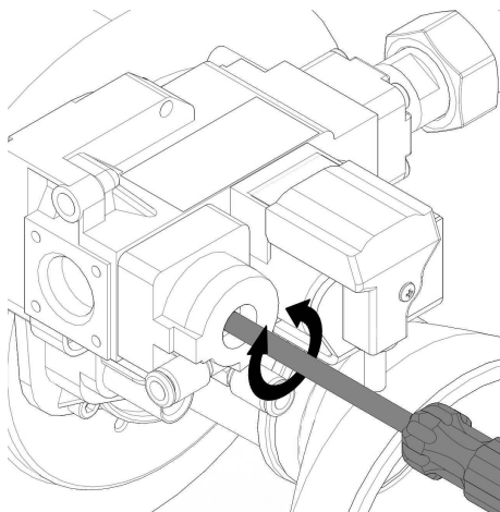
Fig. BFC 28 - 60: ajuste de CO 2 (carga parcial)
