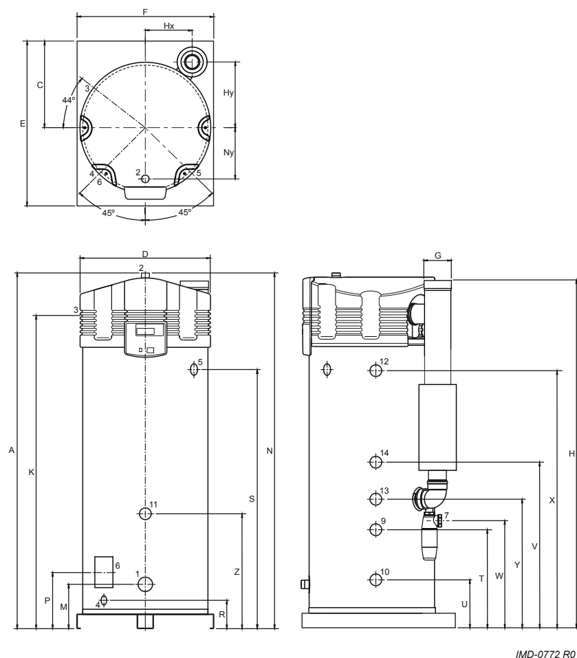
Fig. Dimensiones SGE
