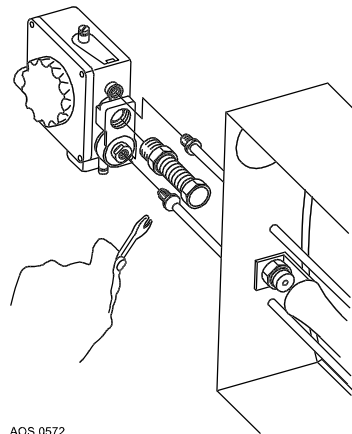
Figure 9 - Démontage brûleur, conduit de la veilleuse et thermocouple
