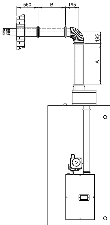
Figure 4 - Dimensions conduit d'évacuation vers mur extérieur
