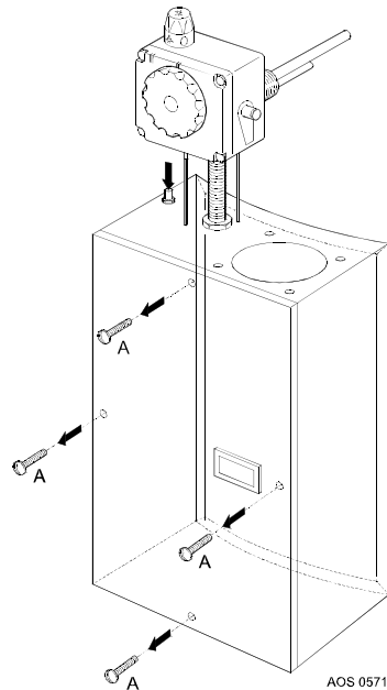
Figure 8 - Démontage chambre de combustion et couvercle
