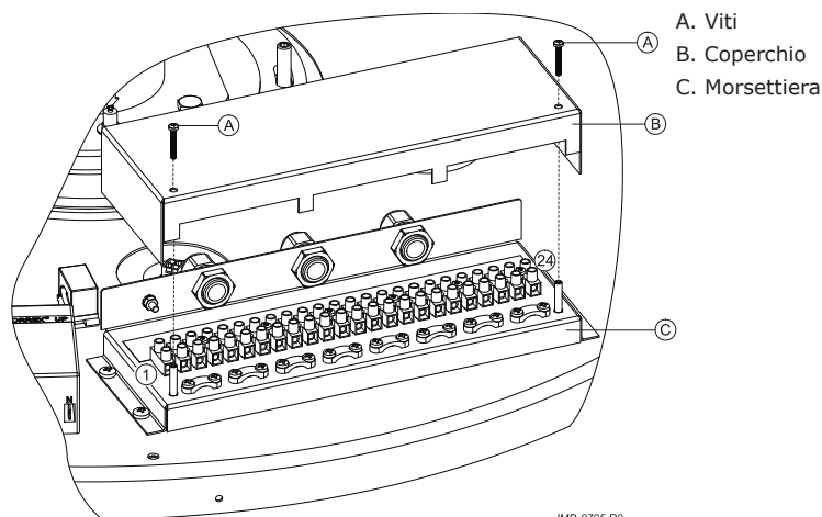
Fig. Morsetteria
