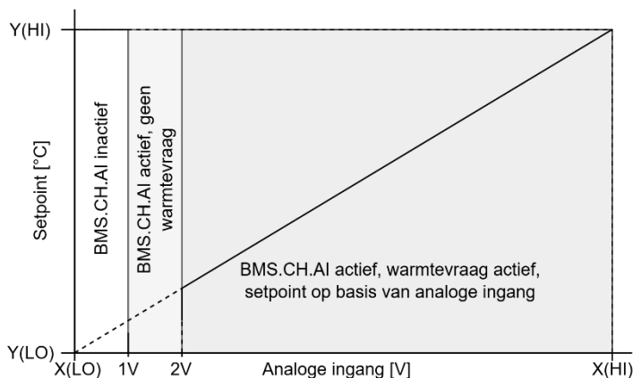
Afbeelding 24 Illustratie van een analoog ingangssignaal voor het gebouwbeheersysteem
