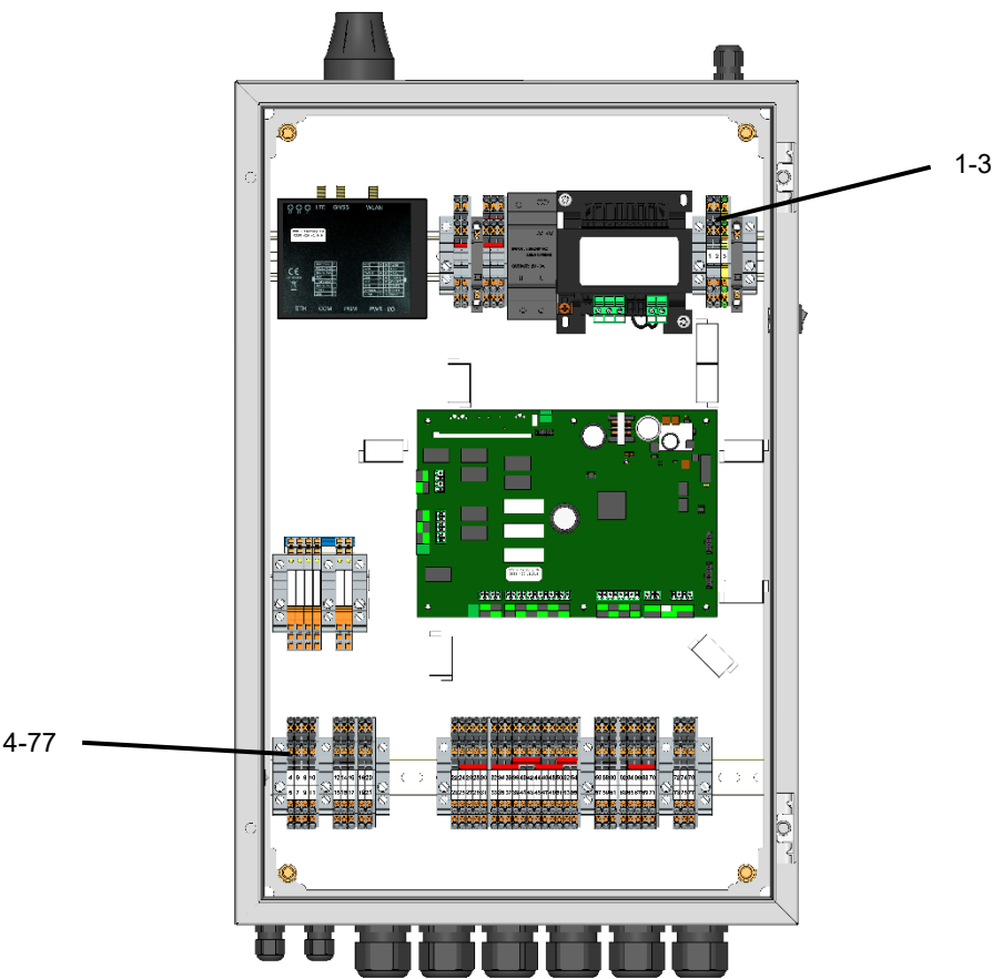
Afbeelding 8 Locatie klemmenstroken
