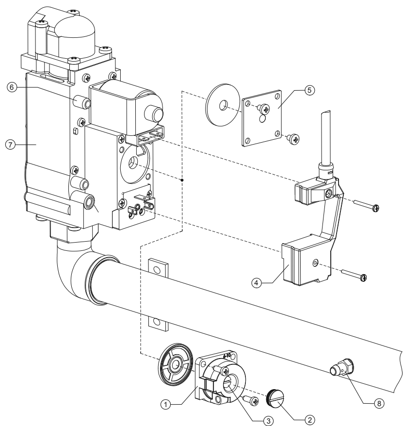
Gasblok voor ADM 40 t/m 115
