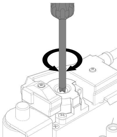
Afb. BFC 80 t/m 120 - CO 2 -afstelling (deellast)
