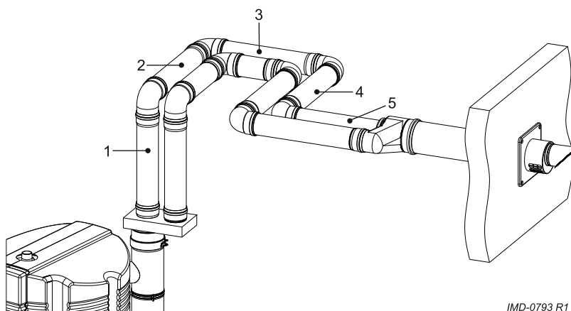
Afb. Voorbeeld van een parallel luchttoevoer- en rookgasafvoersysteem
