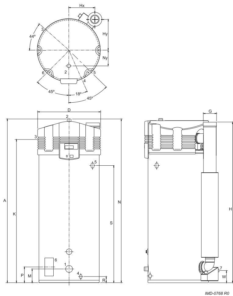
Rys. Wymiary BFC 28, 30, 50, 60
