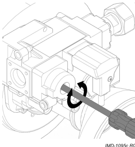
Rys. BFC 80 do 120 — regulacja CO 2 (częściowe obciążenie)
