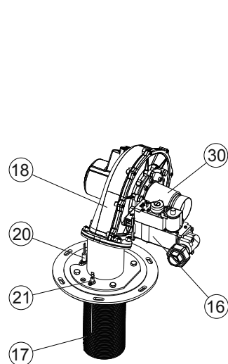
Rys. Podgrzewacz wody BFC 80, 100, 120
