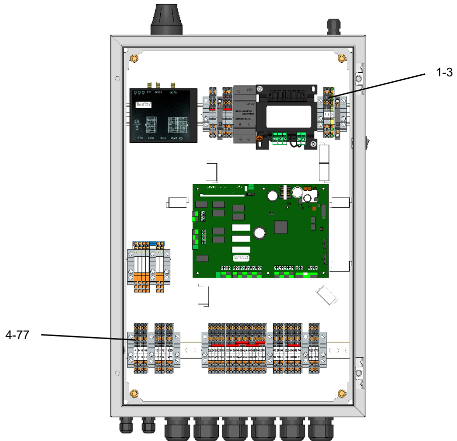
Figure 8 Emplacement des borniers
