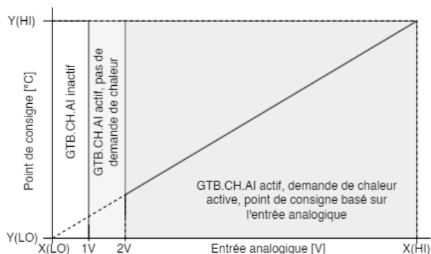
Figure 24 Illustration d'un signal d'entrée analogique pour le système de gestion technique du bâtiment
