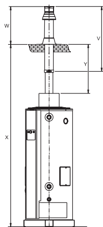
Evacuation coaxiale toiture
