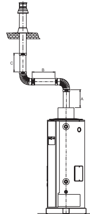
Configuration de la ventouse sortie toiture
