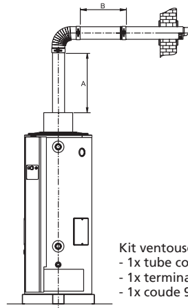
Configuration de la ventouse sortie murale
