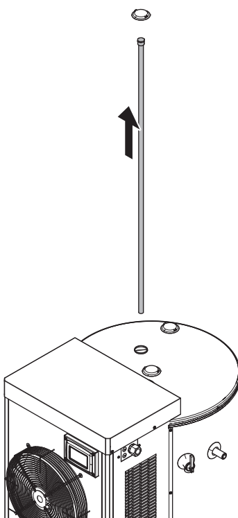
Rys. Sprawdzenie anody
