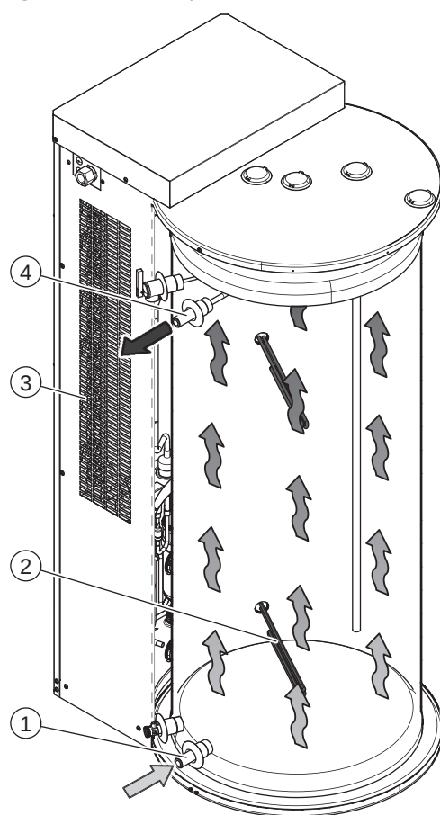
Fig. CAWH scaldacqua
