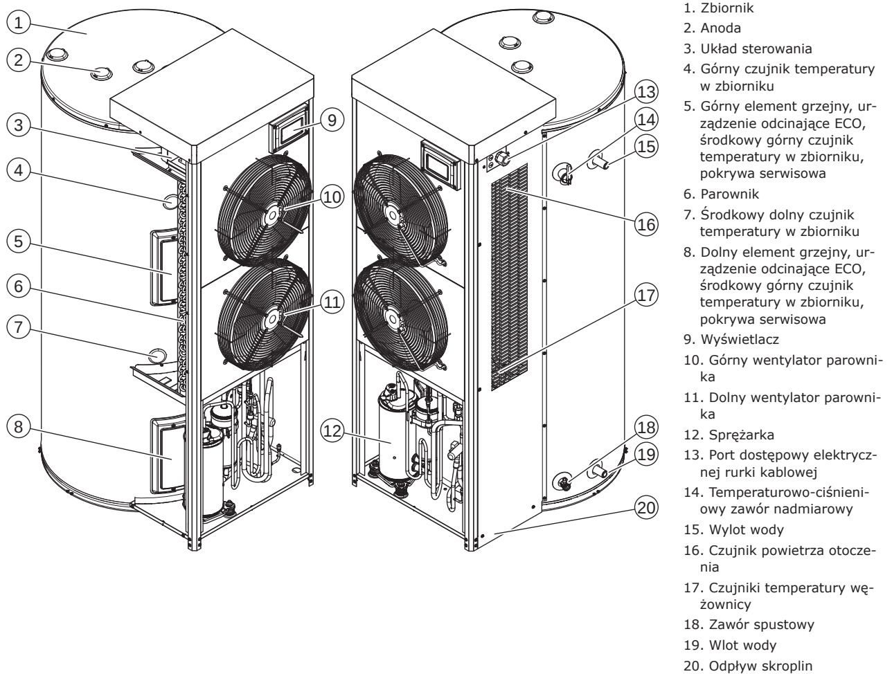
Rys. Elementy podgrzewacza wody
